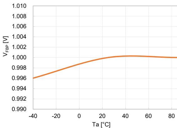
13) V FBP Voltage vs. Temperature V CC = 3.7 V R1287x001y
