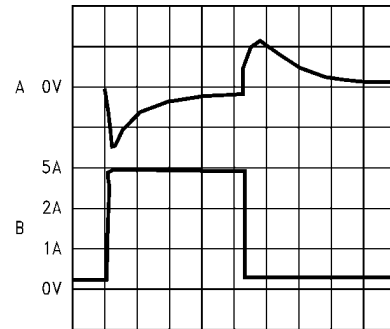
200 \mu sec/Div
