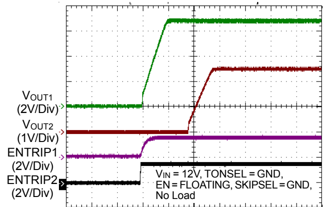
VOUT1 Delay-Start
