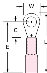
MH18-10R/L Stud Size 10 Wire Range 22-18
