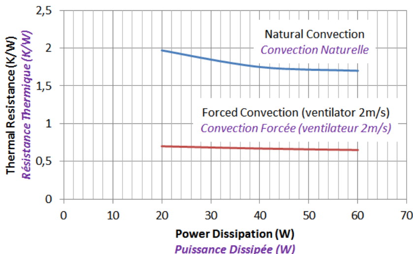
Thermal Resistance vs Power Dissipation Résistance Thermique vs Puissance Dissipée
