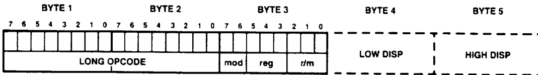
B. LONG OPCODE FORMAT EXAMPLE
