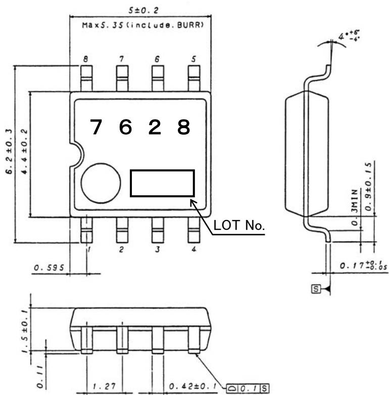
SOP8 ( UNIT:mm )
