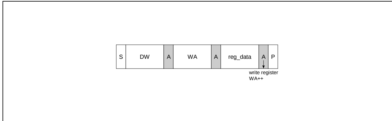
Figure 29. Byte Write
