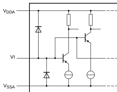
Fig 11. VI analog input
