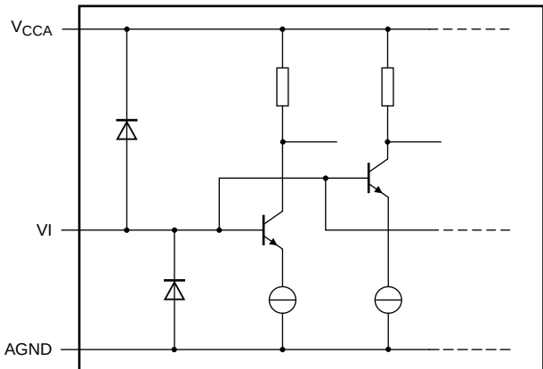
Fig 10. Analog inputs
