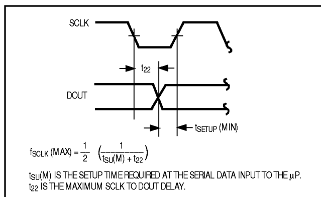
a. SPI b. QSPI c. MICROWIRE d. TMS320 SERIAL INTERFACE
