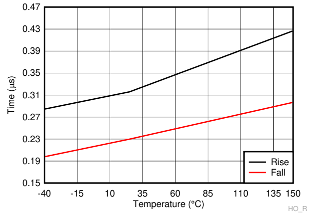
A. C_L=100nF
