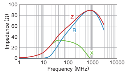
MPZ1005S600CT000
