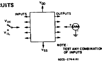
Fig. 10 - Input voltage.
