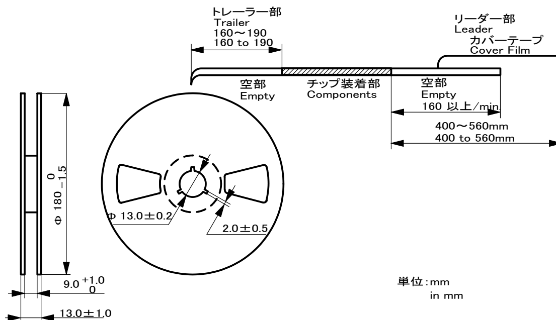
8-2 リール外形寸法図 Dimensions of Reel
