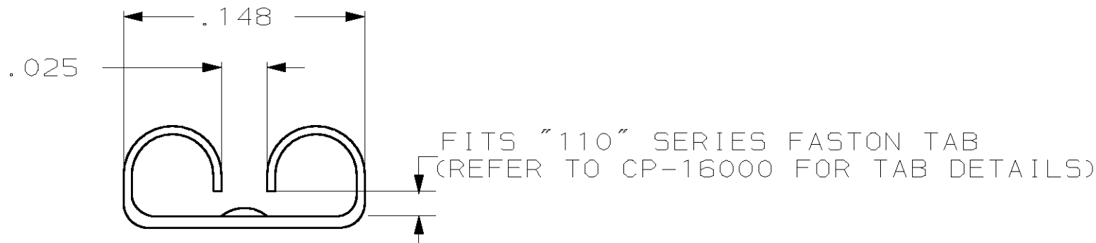
SECT A-A
