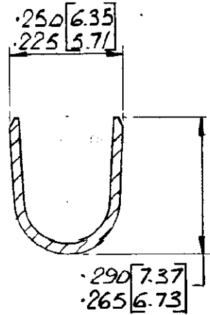
SECTION C-C SCALE: 4:1
