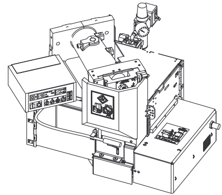
Stripping Module 1490501-[]
