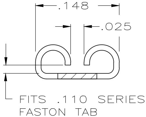
VIEW A-A
