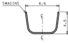
SEC' : C-C"
