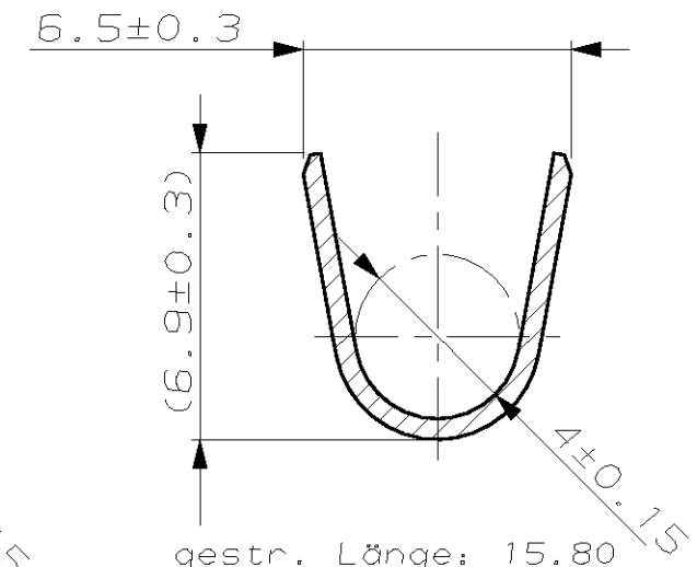
Schnitt: C-C
