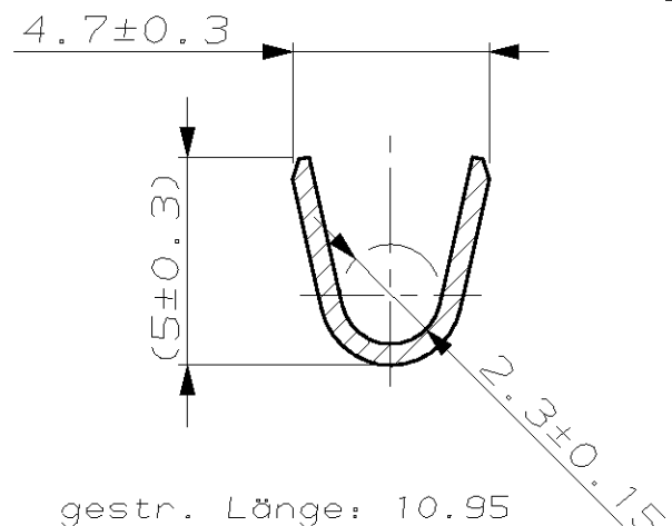
Schnitt: B-B
