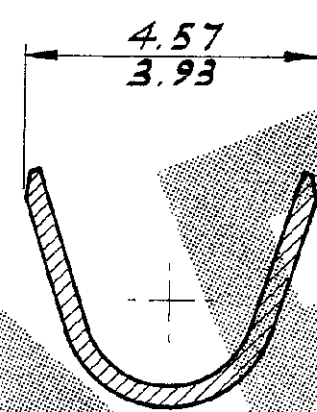
SECTION 'B'- 'B' SCALE 10:1
