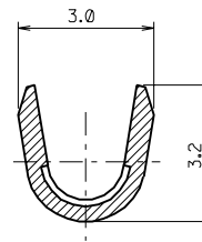
SECTION:C-C*
