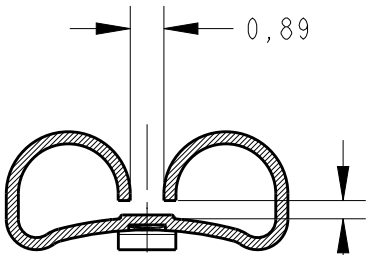
SECTION X-X SCALE 5:1 PARA LINGUETA DE 0,8mm ESPESSURA
