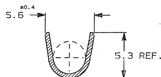
SEZIONE B-B (SECTION B-B)
