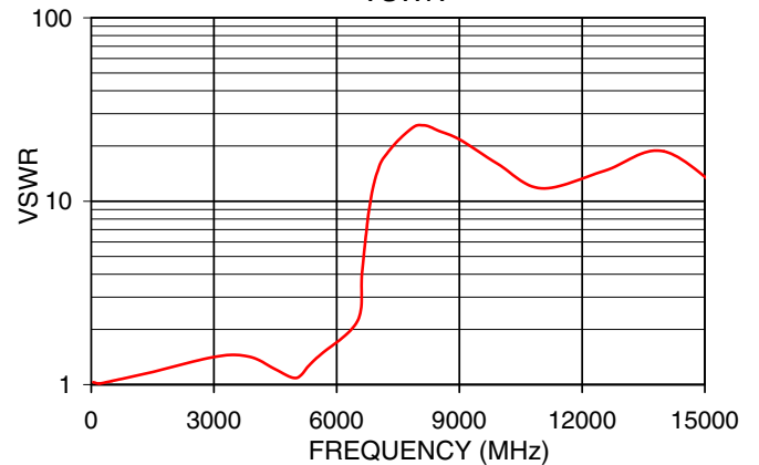
LFCN-5850D+ VSWR
