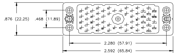
56 PIN RECEPTACLE
