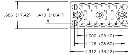
20 PIN RECEPTACLE
