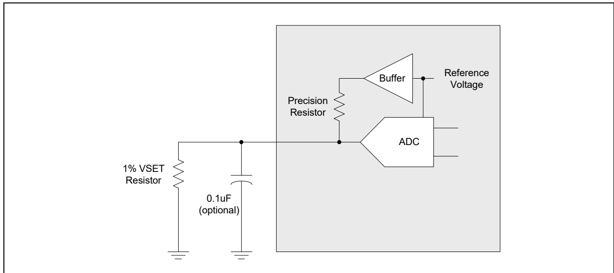
FIGURE 38-6: VSET CIRCUIT
