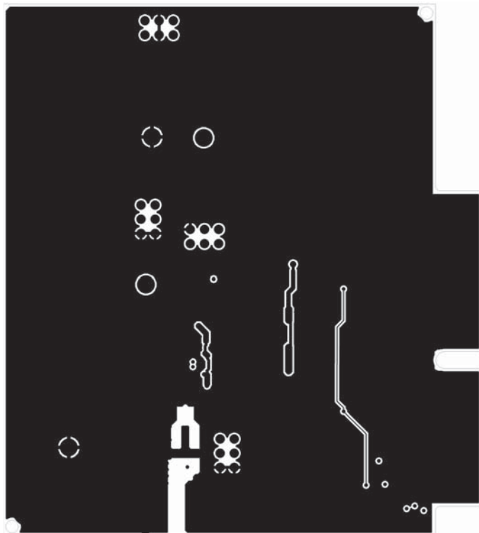
Layer 5 GND
