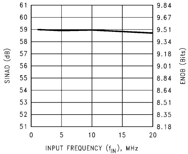
SINAD & ENOB vs. f_{IN}
