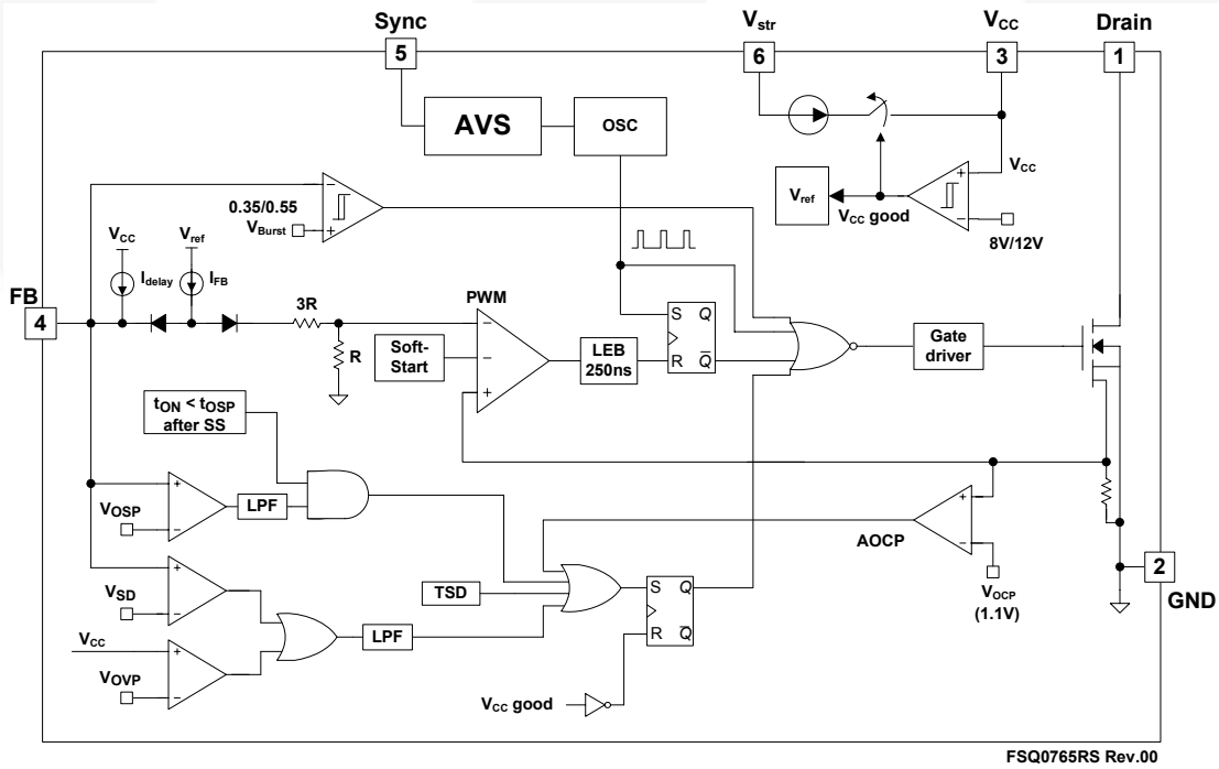
FSQ0765RS Rev.00
