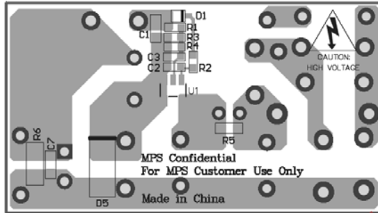
Bottom layer
